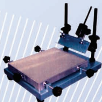
▲ WSC-200H ΧΕΙΡΟΚΙΝΗΤΗ ΕΠΙΠΕΔΗ ΜΗΧΑΝΗ
